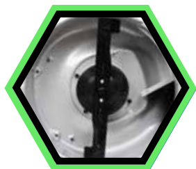
Lame à 2 dents pour la coupe et le mulching.
